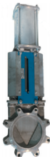
Full Lug model
